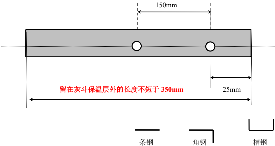
安装示意图
